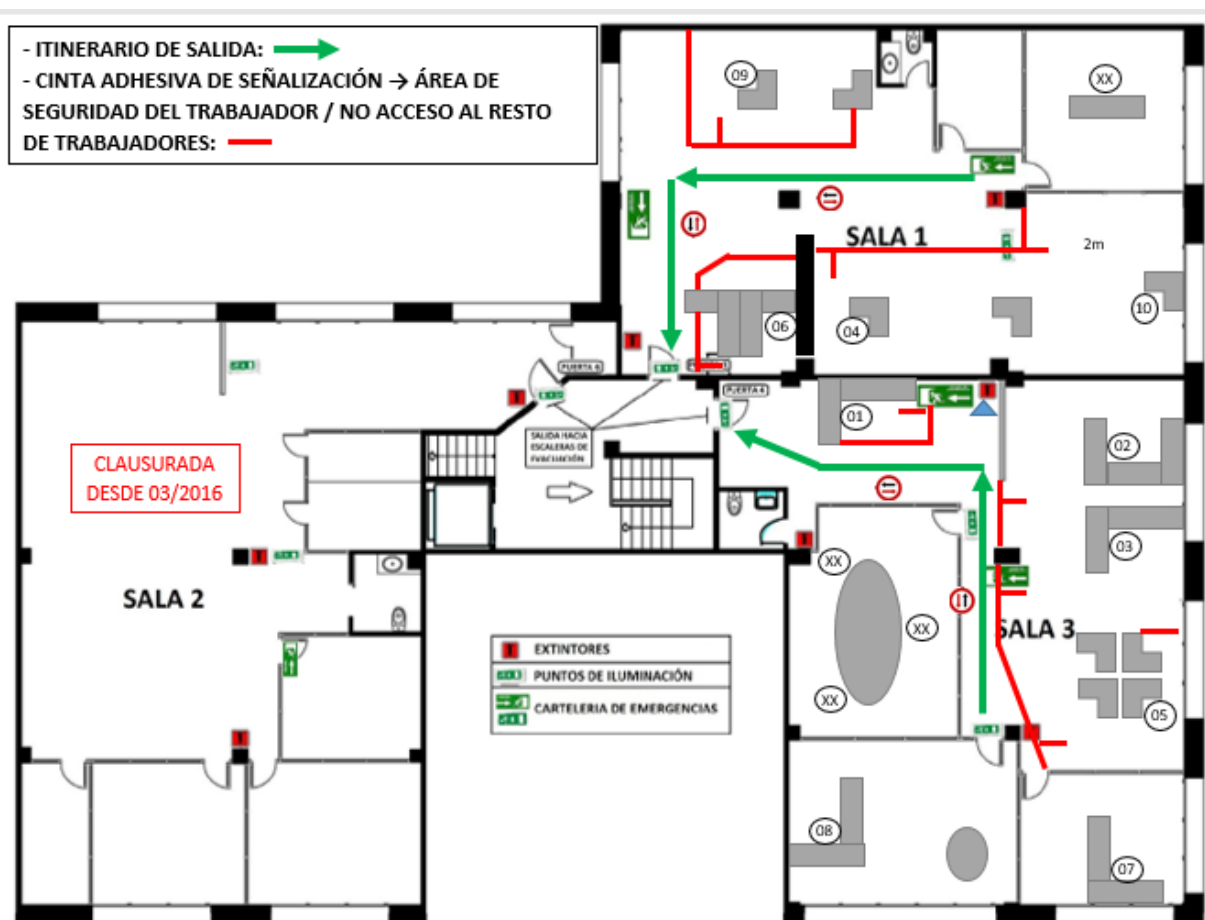
PLANO DE EMERGENCIAS - OFICINAS
